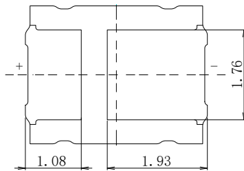
1-3 Bottom view 背视图
