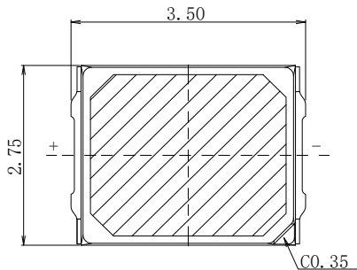
1-1 Top view 正视图
