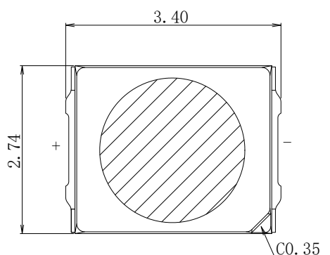
1-1 Top view 正视图
