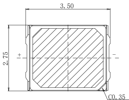
1-1 Top view 正视图
