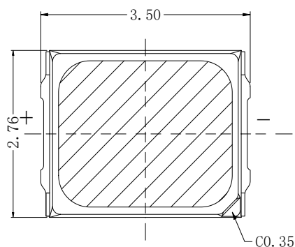
1-1 Top view 正视图
