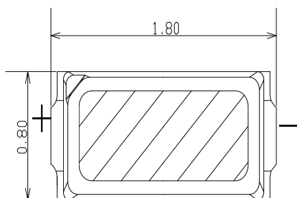
1-1 Top view 正视图
