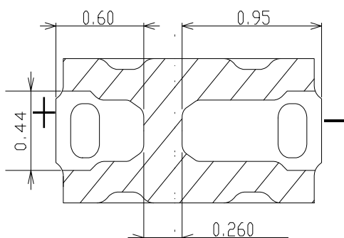
1-3 Bottom view 背视图
