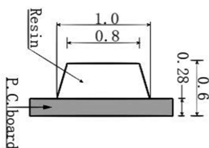
1-2 Side view侧视图
