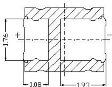
1-3 Bottom view 背视图
