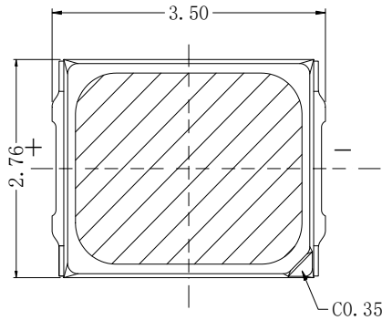
1-1 Top view 正视图
