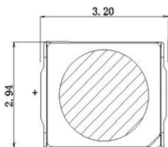
1-1 Top view 正视图
