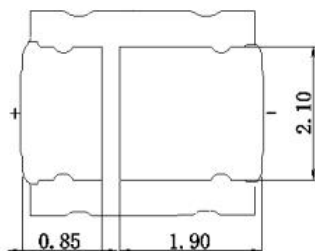
1-3 Bottom view 背视图
