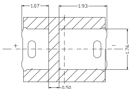
1-3 Bottom view 背视图
