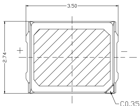
1-1 Top view 正视图
