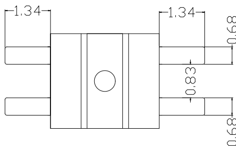
1-3 Bottom view 背视图
