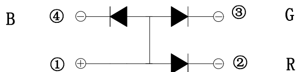
1-5 Polarity 极性
