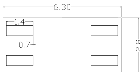
1-3 Bottom view 背视图
