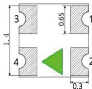
1-3 Bottom view 背视图
