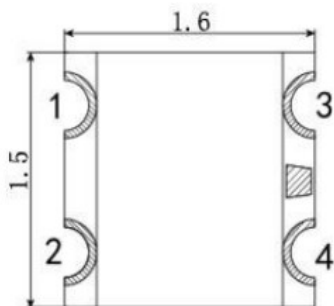
1-1 Top view 正视图
